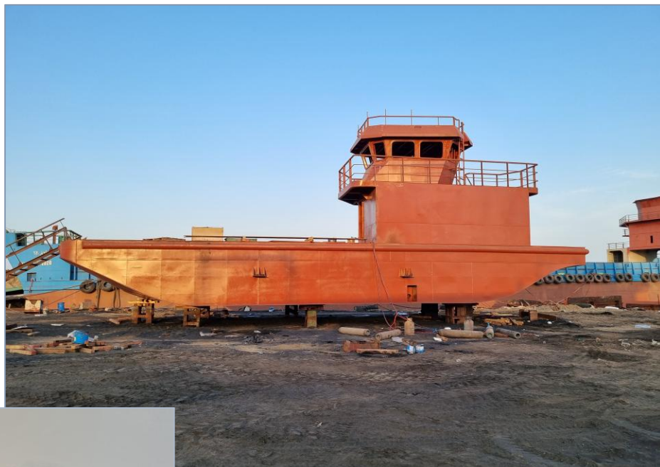
شناور مولتی کت در حال ساخت: مدل ZHIK 1
